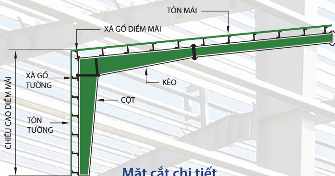
Mặt cắt chi tiết
